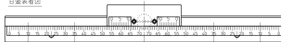
目盛装着図
