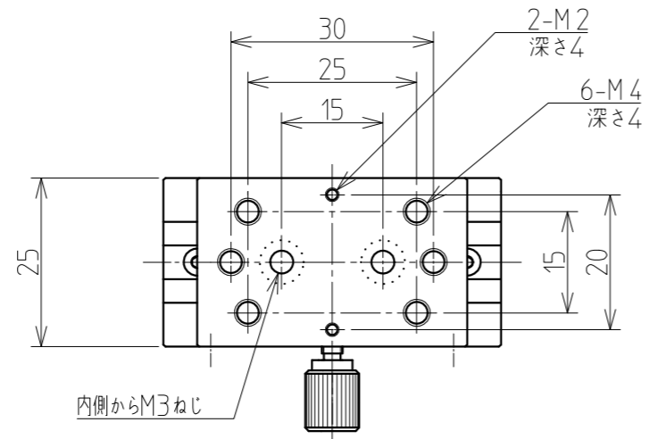
目盛装着図
