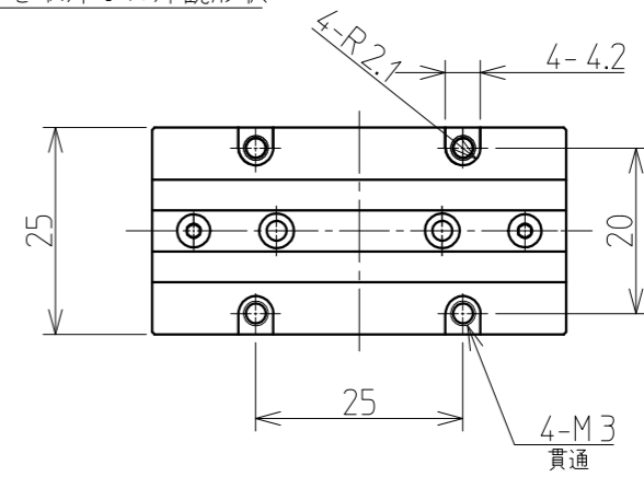
可動部を取外した外觀形状
