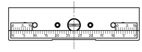
目盛装着図
