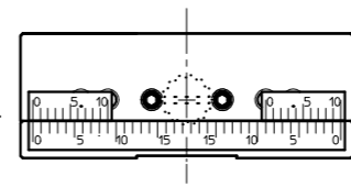
目盛装着図
