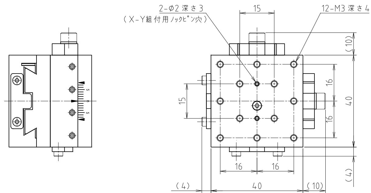
上面
