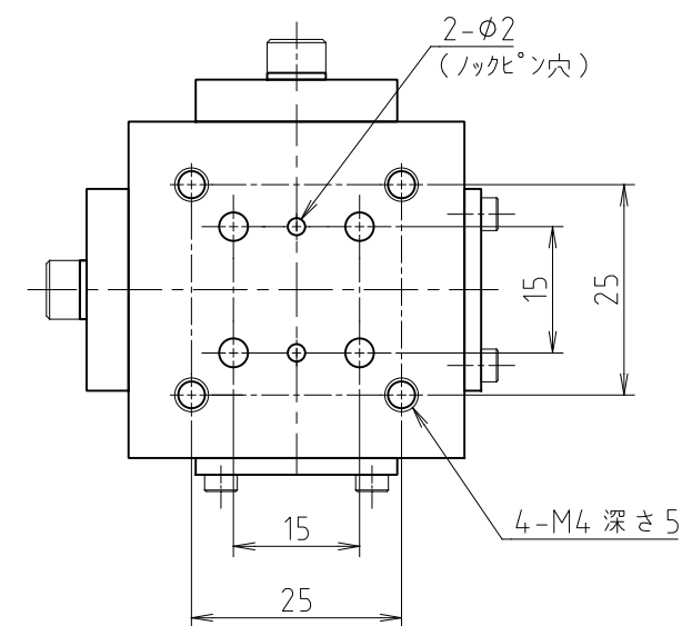
底面
