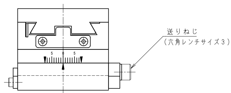
上面
