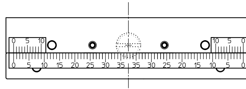
目盛装着図
