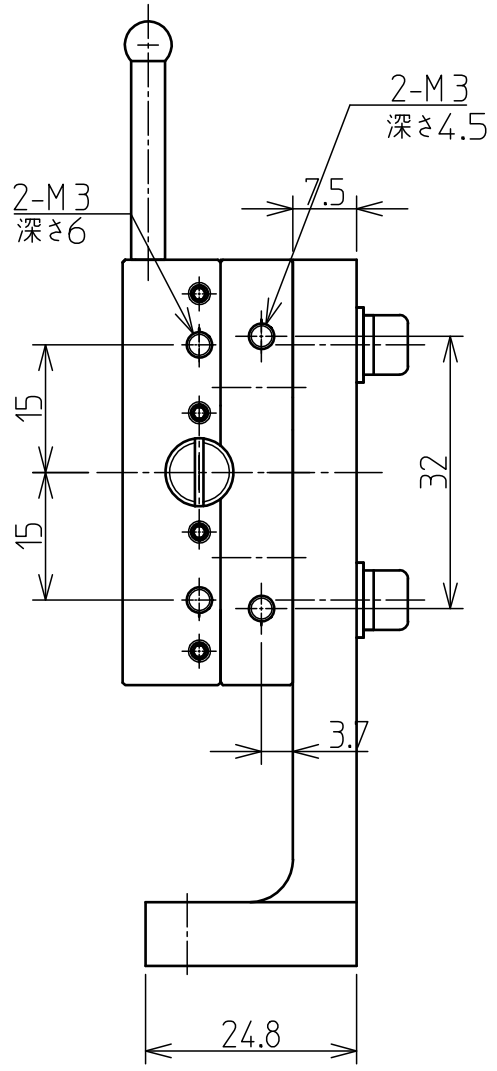
目盛装着図
