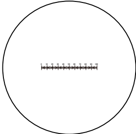
10mm100等分目盛(最小目盛0.1mm)
