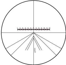
12mm120等分目盛(最小目盛0.1mm) 十字線、55°、60°、90°、120° 角度線
