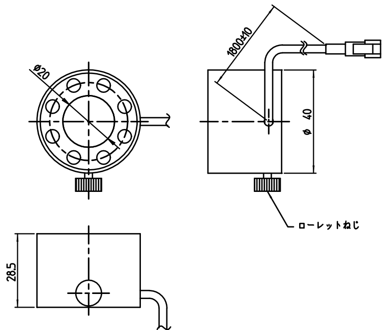
ML-8 用LED照明部
