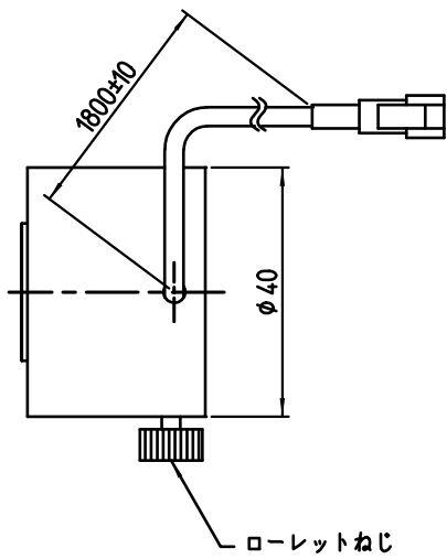
ML-TV6LED照明部
